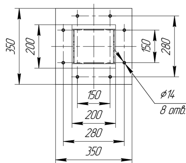
В(1:10) 4 места
