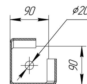
Г-Г(1:5) 16 мест
