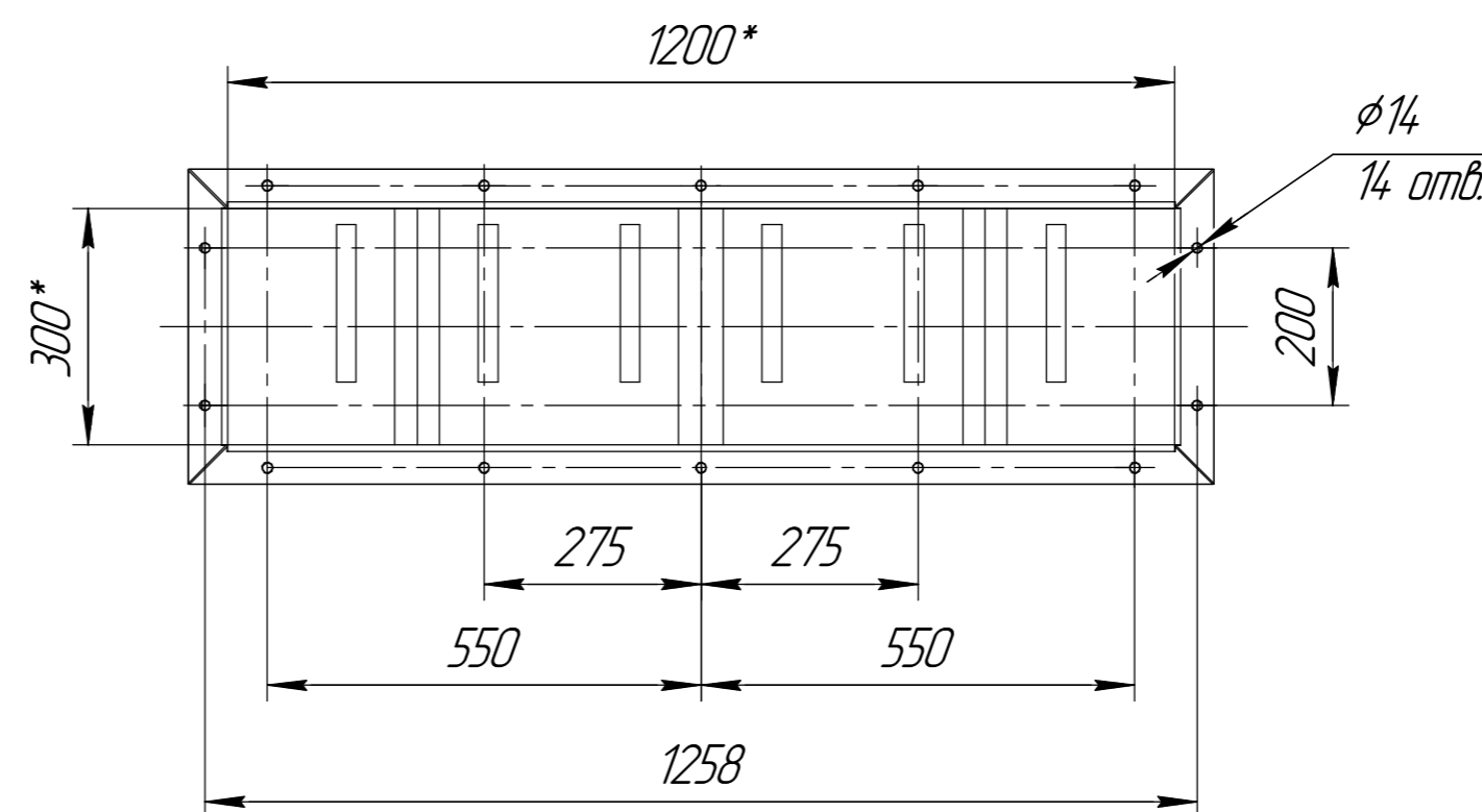
A(1:10) 2 места
