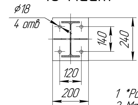
В-В(1:10) 10 мест
