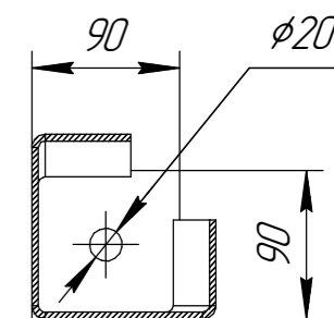
Г-Г(1:5) 4 места
