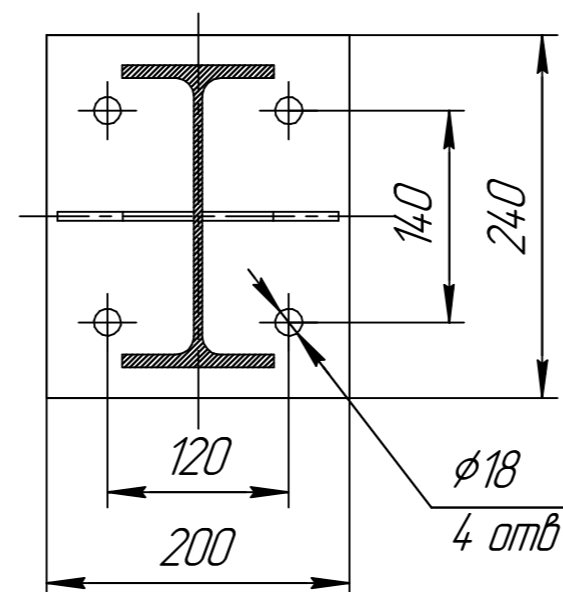
В-В(1:5) 12 мест
