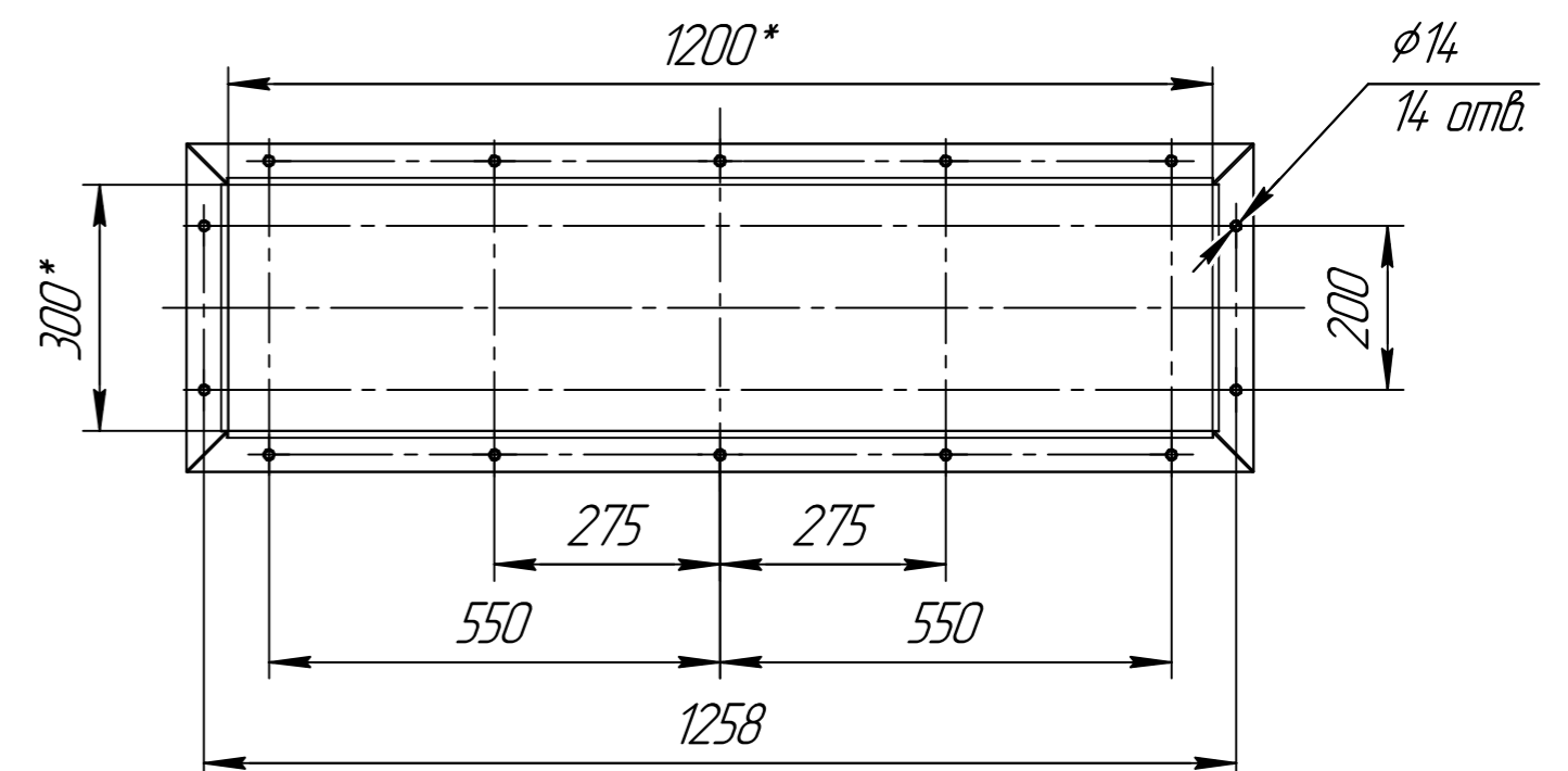
А,Б(1:10)
