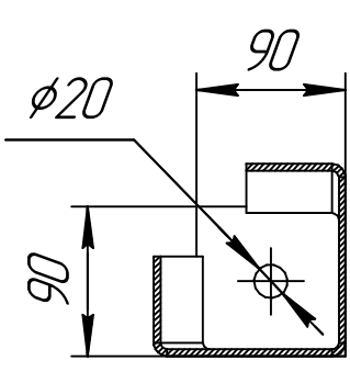
В-В(1:5) 16 мест
