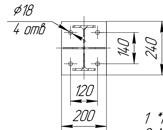
В-В(1:10) 10 мест
