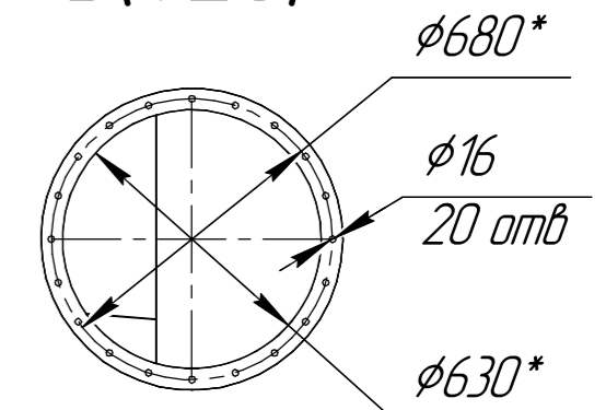
Б(1:20)
