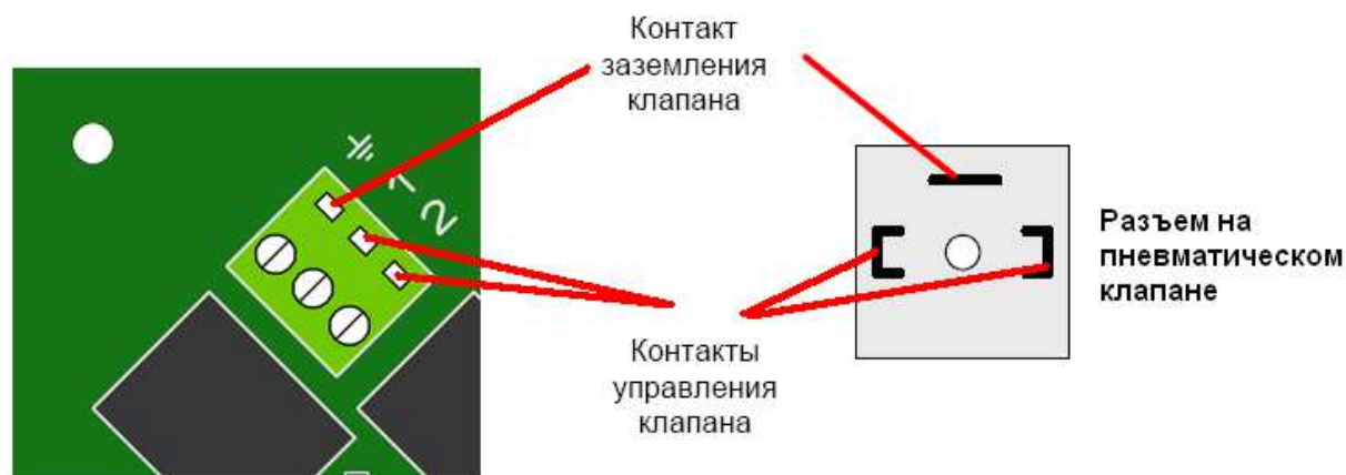
Рис. 4 – Подключение клапанов.
