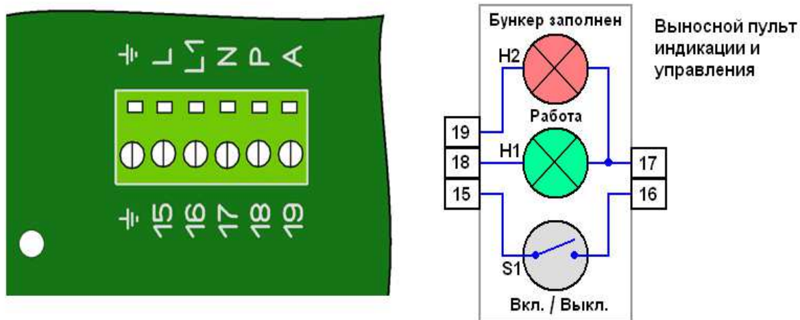
Рис. 5 – Подключение пульта.
